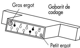
Résultat du perçage
